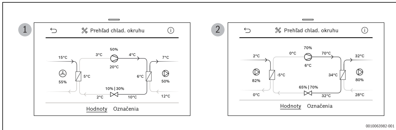
Obr. 7 Prehľad chladiaceho okruhu
