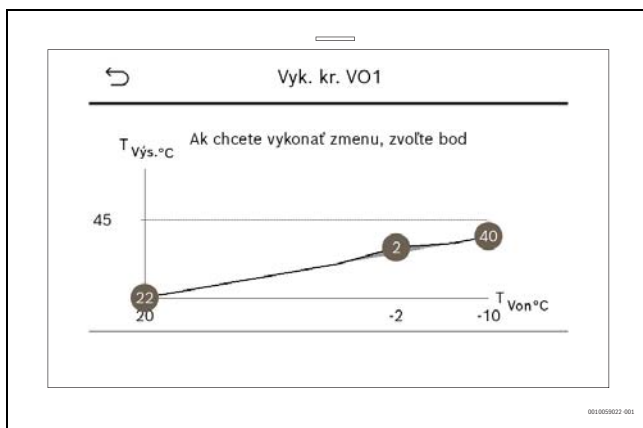
Obr. 1 Úvodná obrazovka na nastavenie vykurovacej krivky pre typ regulácie vonkajšej teploty pomocou päťm bodu (a komfortného bodu)
