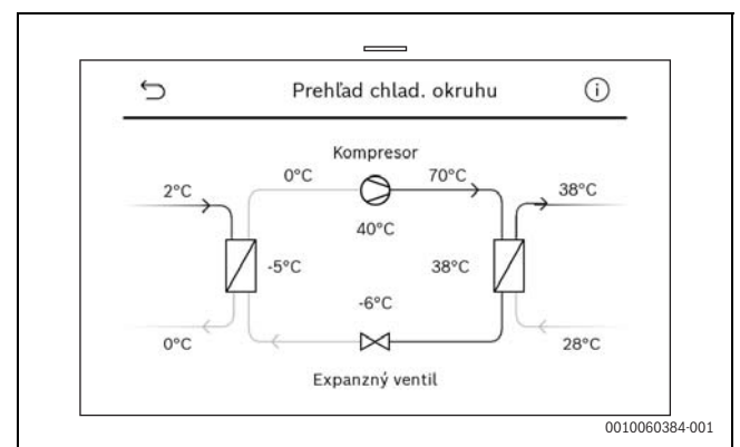
Obr. 10 Prehľad chladiaceho okruhu
