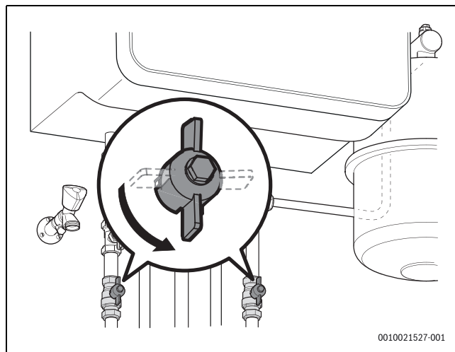
Obr. 3 Kohút výstupu a spiatočky vykurovania (príklad)
