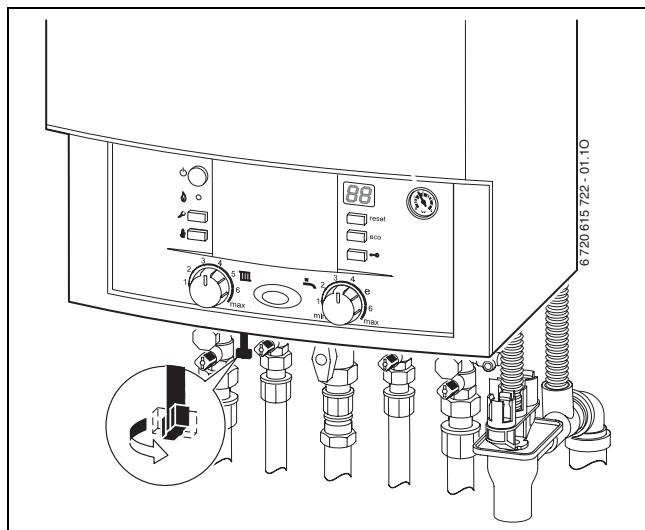
Obr. 11 Montážna pripojovacia doska (vertikálne pripojenie)
