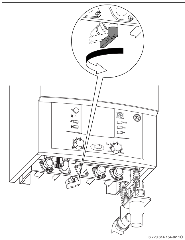
Obr. 3 Montážna pripojovacia doska (vertikálne pripojenie)
